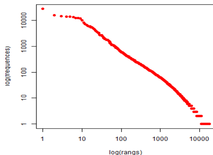
Figure 1 : Distribution des formes lexicales du corpus selon la loi de Zipf
