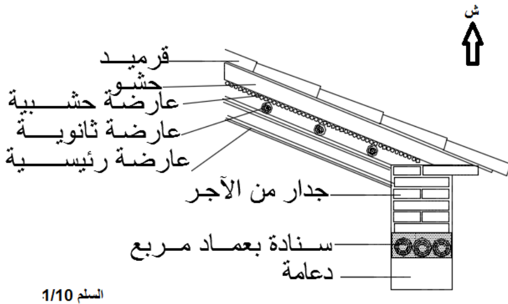
شكل (07): رفع لطريقة التسقيف بالخشب (عن الطالبة)
