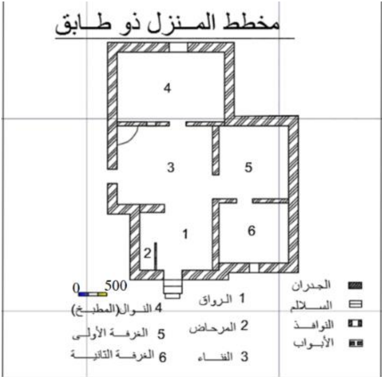
مخطط (14):المنزل ذو طابق
