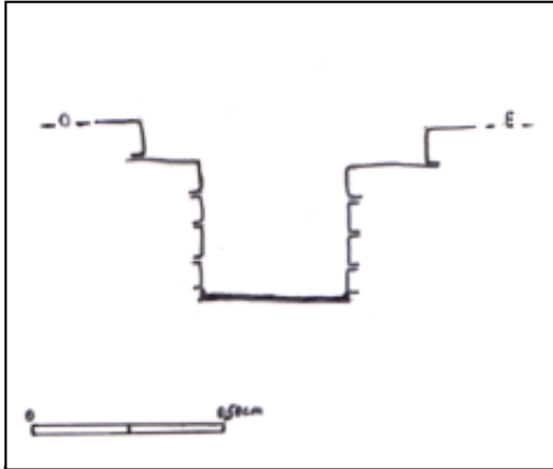
الشكل 20-21 مقطع عرضي لنفس المدفن
