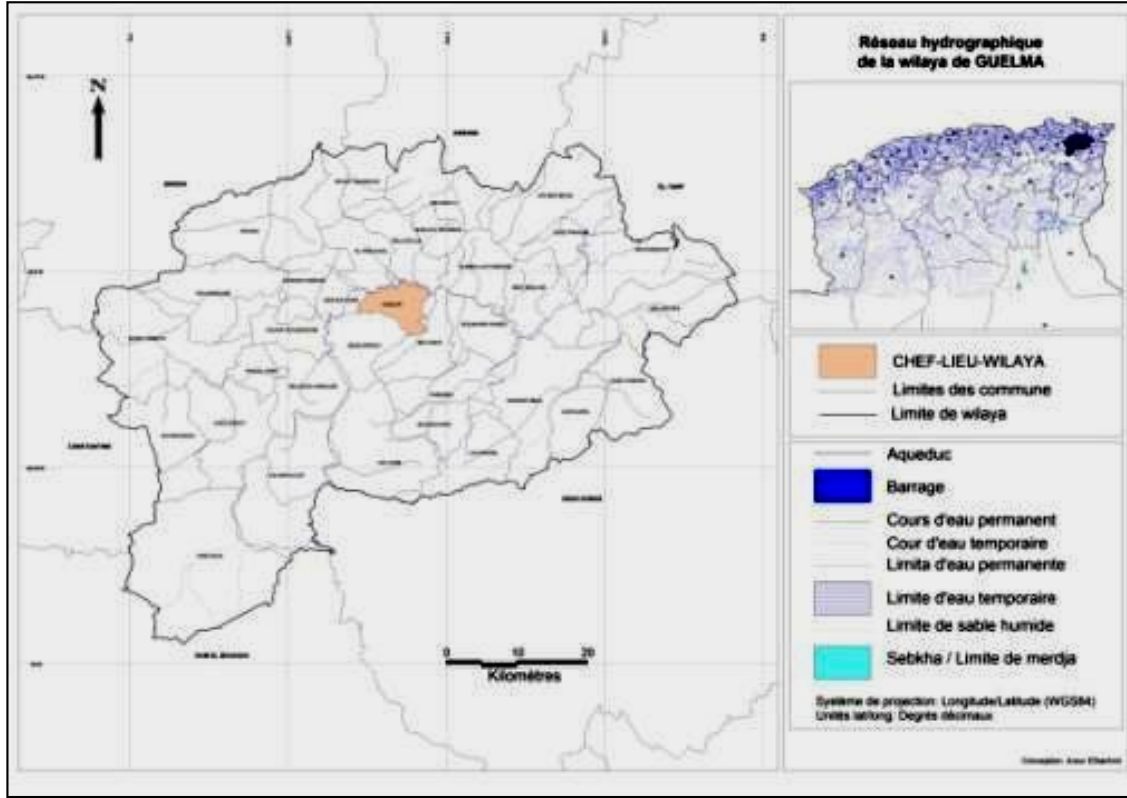
الشكل 3: شبكة المجاري المائية لولاية قالمة Google maps
