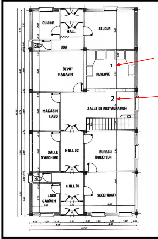
المخطط رقم 2 : الهيكل الإداري للمتحف (بتصرف الطالب) سلم: 100/1
