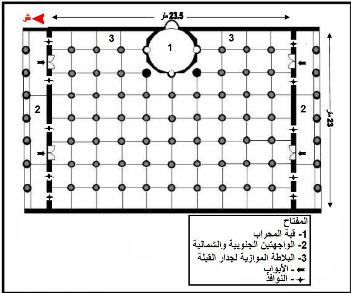
(الشكل رقم 26) المخطط الحالي لجامع سوق الوادي
