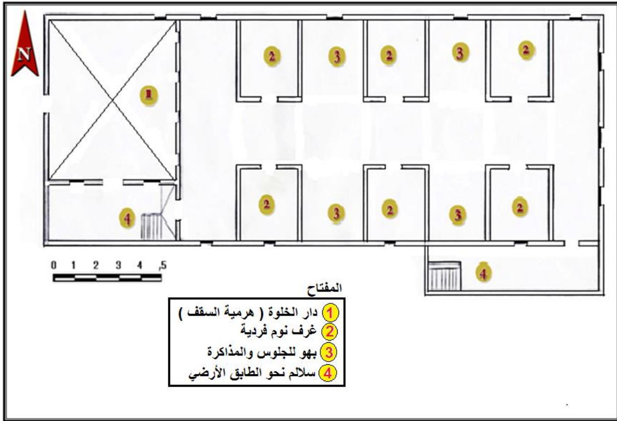
( الشكل رقم 31 ) مخطط القاعة الهرمية بالزاوية التيجانية بقمار
