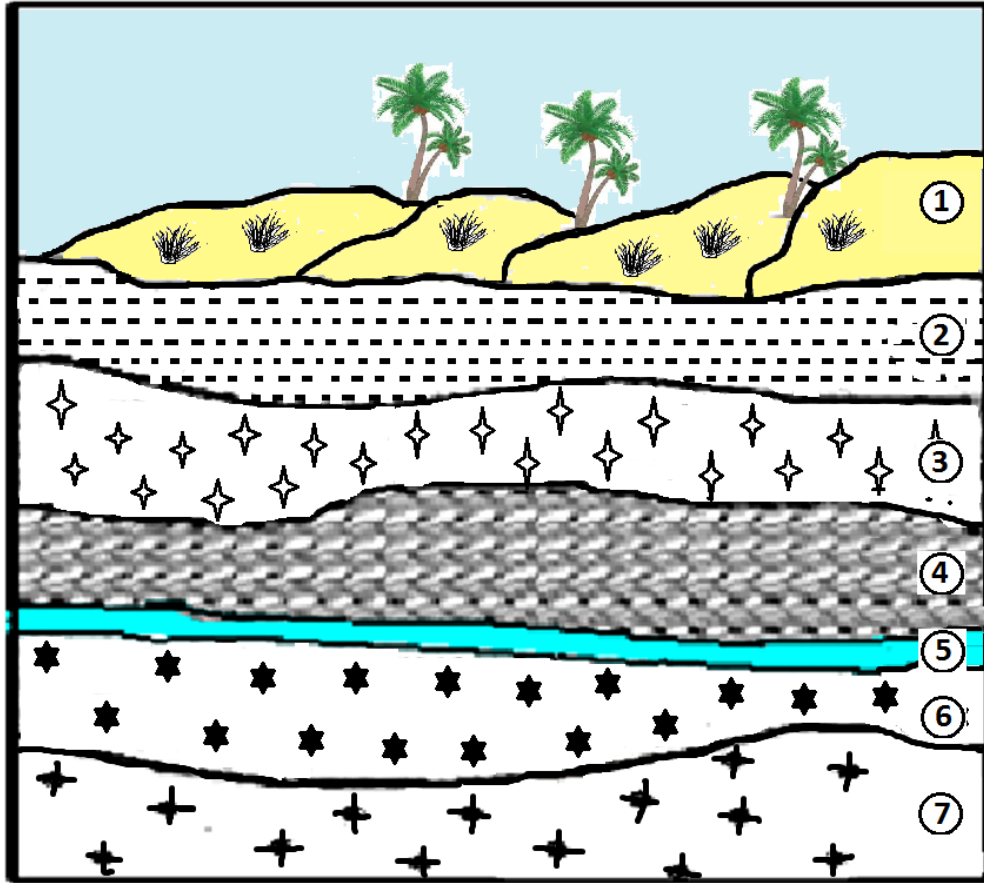
1- كتبان رملية 2- رمال وترشة 3- طبقة حجارة اللوس 4- طبقة حجارة التآفة 5- طبقة الصلصلة 6- رمل ذو مكونات معدنية 7- الحوض المائي
