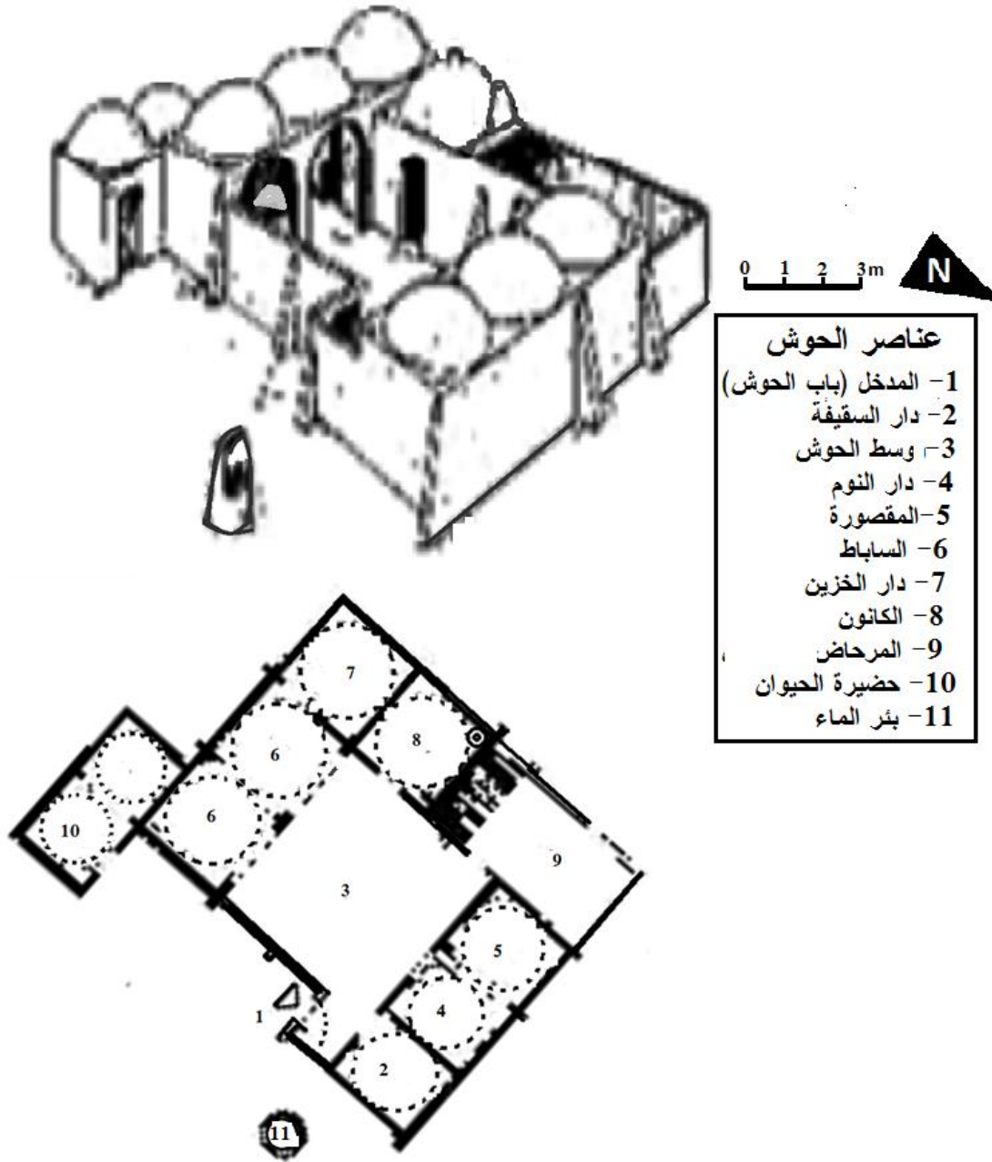
(الشكل رقم 34) مخطط نموذجي للحوش في منطقة سوف
